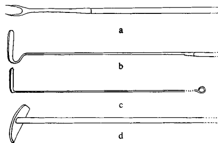
Kachelgereedschap: a. stookgaffel; b. en c. rakelijzers; d. astrekker
